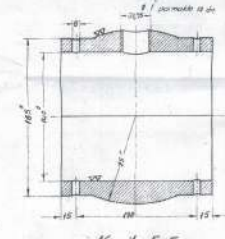
Kesit E-F
