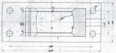
Kesit A-B
