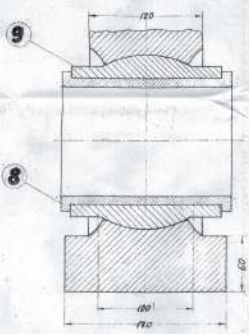
Kesit C-D
